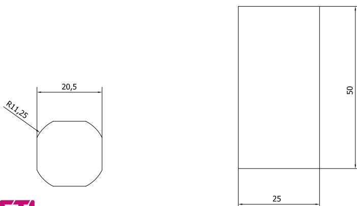
Door drilling
