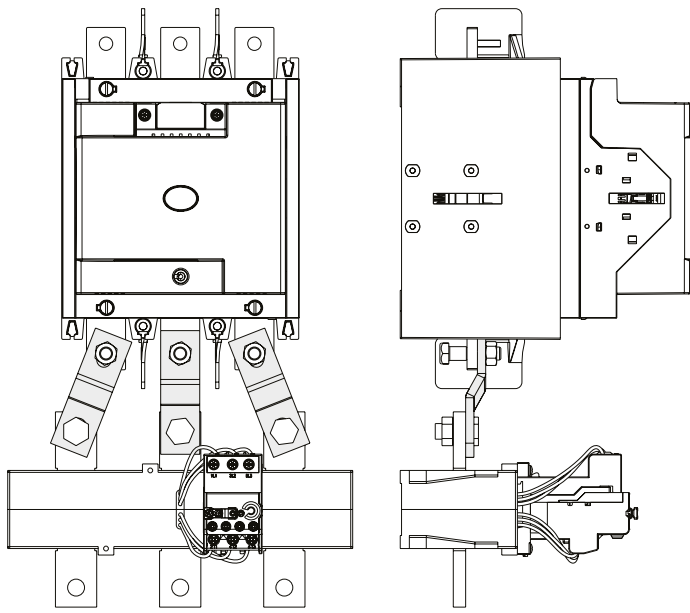
CEM450E/560E + RE407D (400...600A)
