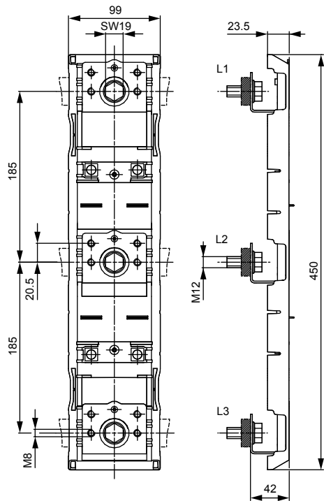
adapter DA 185-185/42
